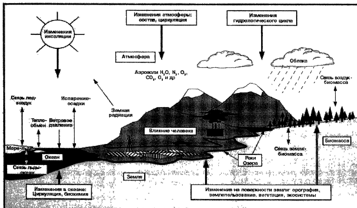
Схематическое изображение климатической системы
