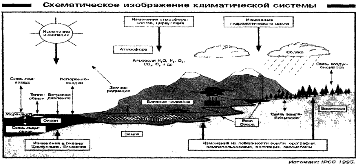
Рисунок 1 – Схематическое изображение климатической системы
